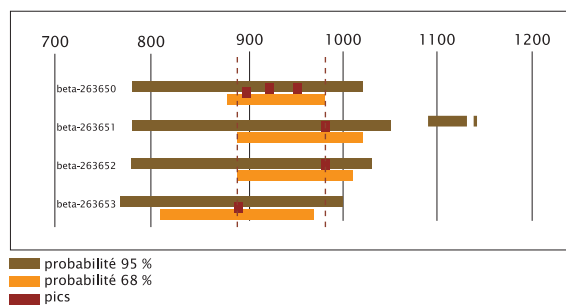
Fig. 6. La chronologie de l'activité sidérurgique d'après les résultats des datations 14C réalisées dans les ferriers de la ZAC.
